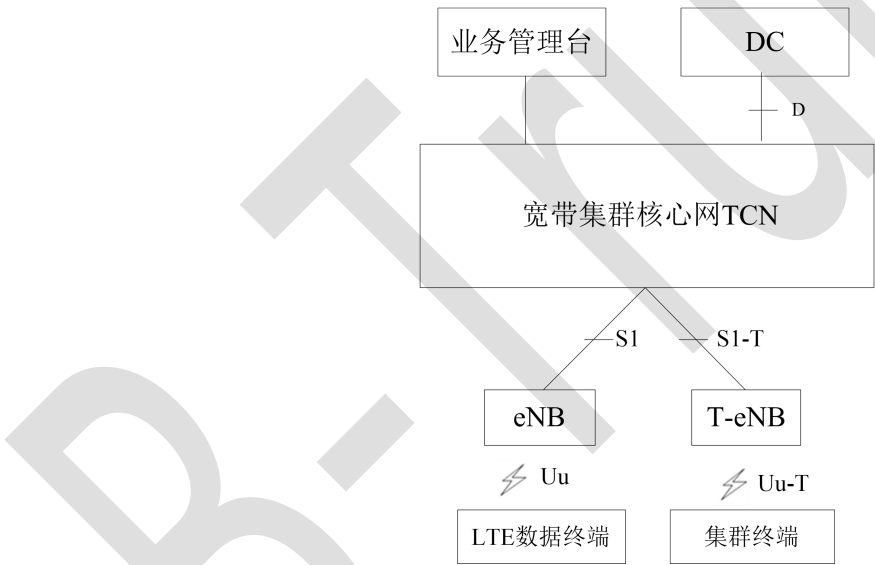
图 1 基于 LTE 的宽带集群系统架构
